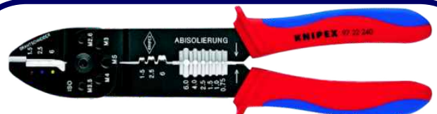
Lisovacie kliešte Obj. č. 97 22 240
